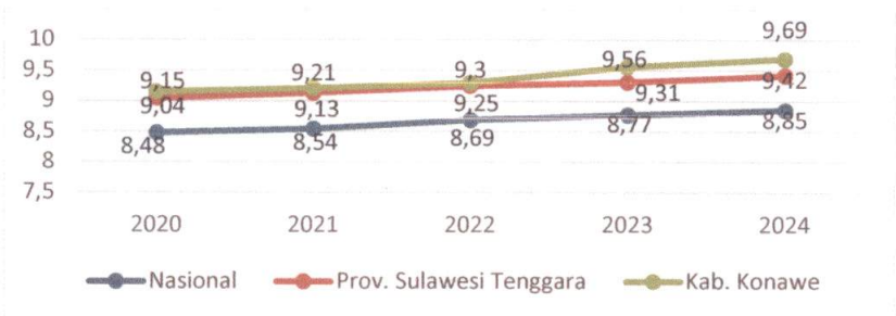
Gambar 2. 9 Perbandingan Capaian Rata-Rata Lama Sekolah Antara Kabupaten Konawe, Provinsi Sulawesi Tenggara, dan Nasional Tahun 2020-2024
